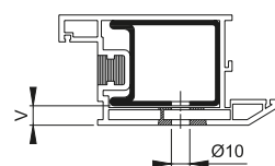
kunststof-profiel
