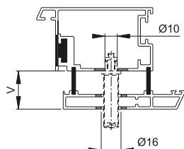
aluminium-profiel
