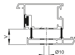
aluminium-profiel
