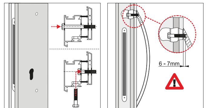
Montagevoorbeeld
