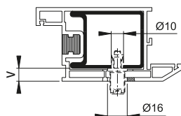
kunststof-profiel
