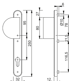
Verkropte greep 554
