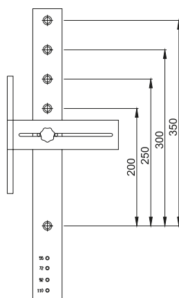
boormal voor beugelgrepen
