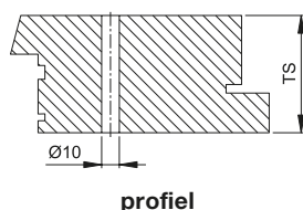
profiel
