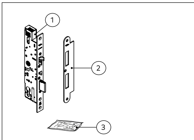
Afb. 3 Meegeleverde onderdelen
