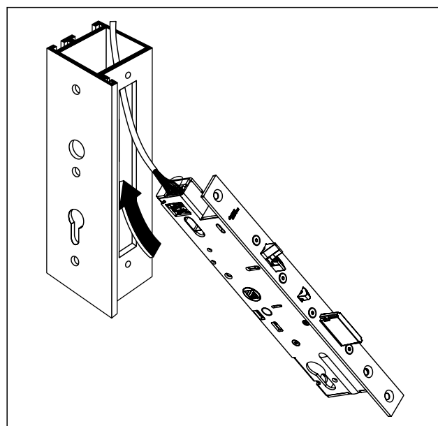
Afb. 16 Anti-paniekslot aanbrengen
