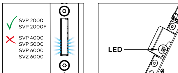
Afb. 29 Ledweergave in de schoottuitsparing voor sloten voor volbladdeuren
