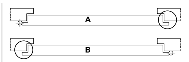
Afb. 7 Vouwdeuren
