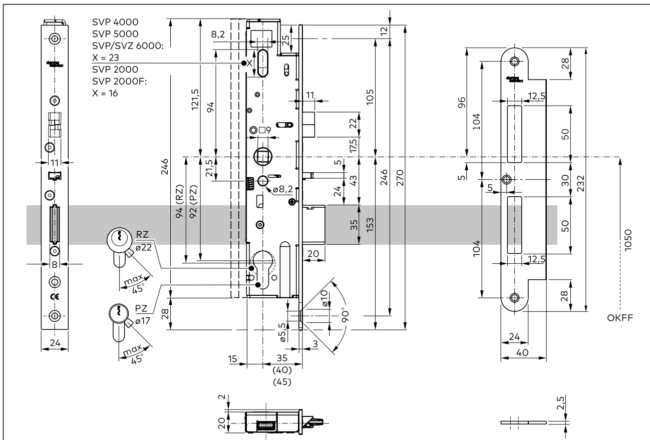
Afb. 4 Slotafmetingen
