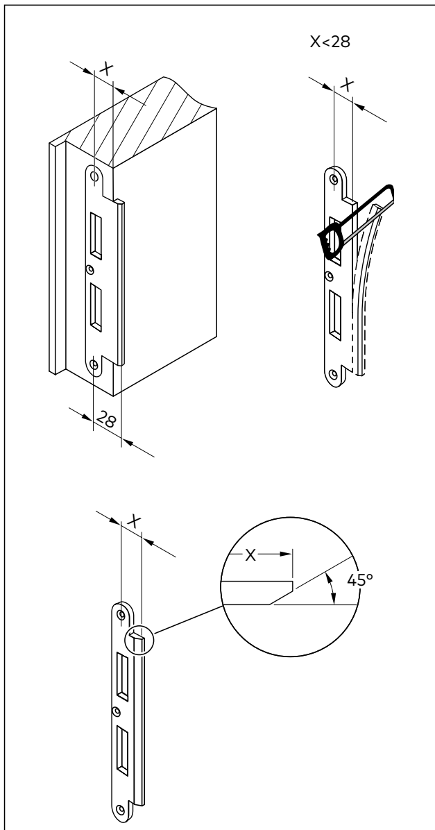
Afb. 26 Maten van de aanpassingen
