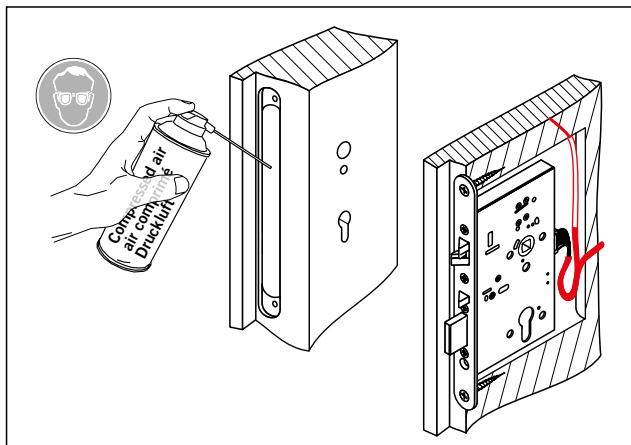
Afb. 23 Anti-paniekslot aanbrengen
