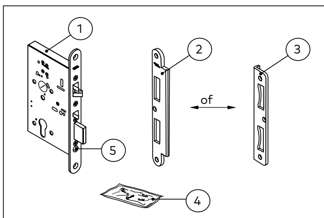
Afb. 5 Meegeleverde onderdelen
