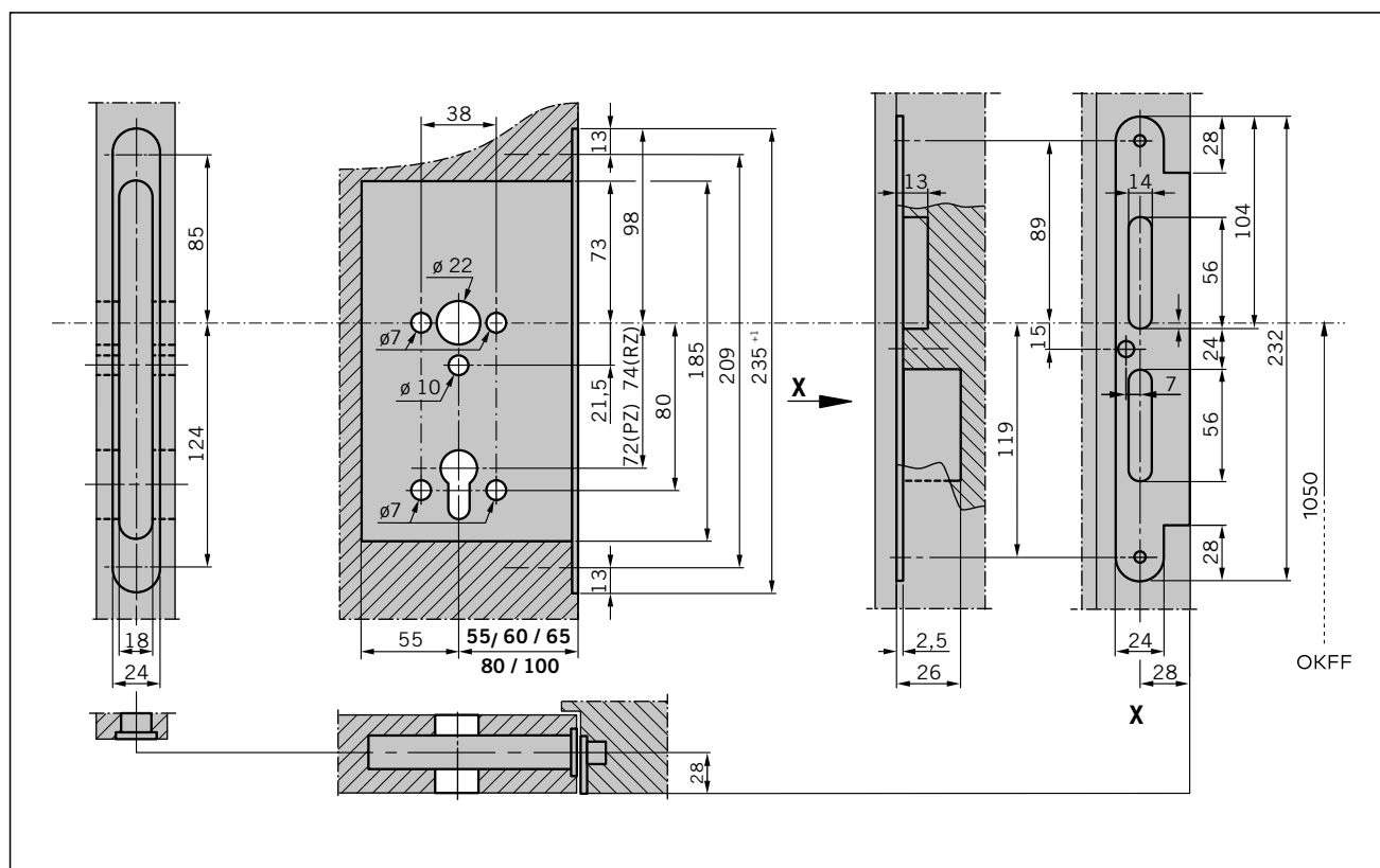
Afb. 13 Uitsparingen en voorgeboorde gaten in het deurblad en het deurkozijn met een sluitplaat met lip
