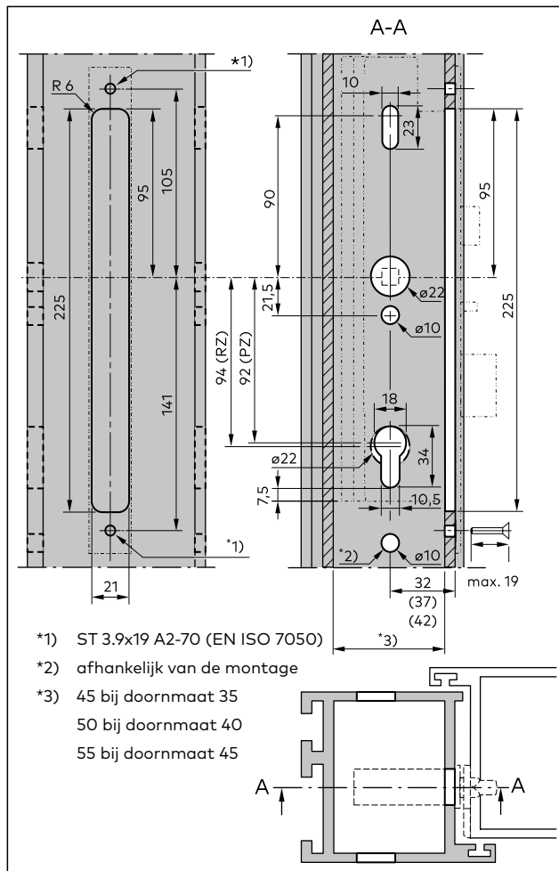
Afb. 10 Uitsparingen en voorgeboorde gaten in het deurblad
