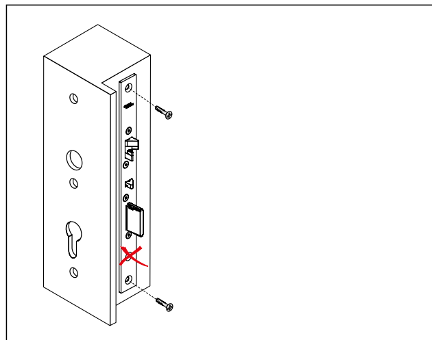
Afb. 24 Anti-paniekslot vastschroeven.
