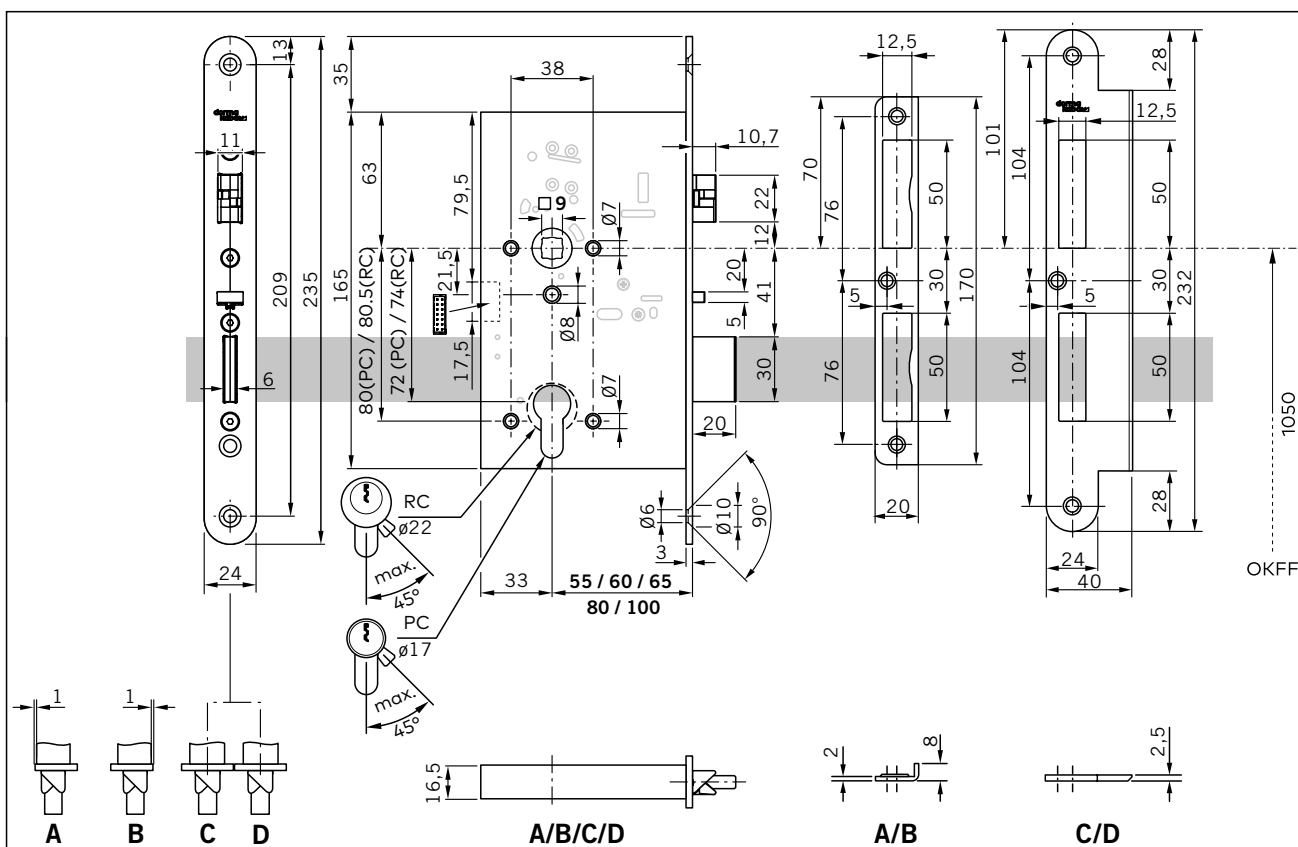
Afb. 6 Slotafmetingen
