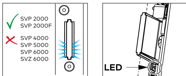
Afb. 28 Ledweergave in de schoottuitsparing voor profiel-slotten
