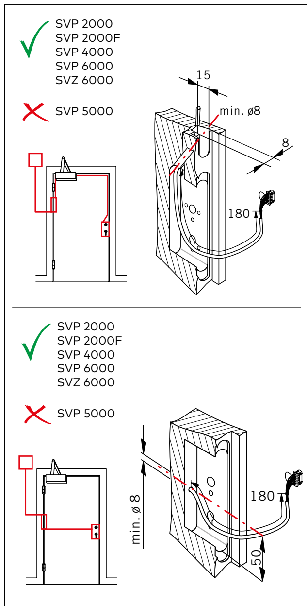
Afb. 14 Uitsparingen en voorgeboorde gaten in het deurblad voor bedrading
