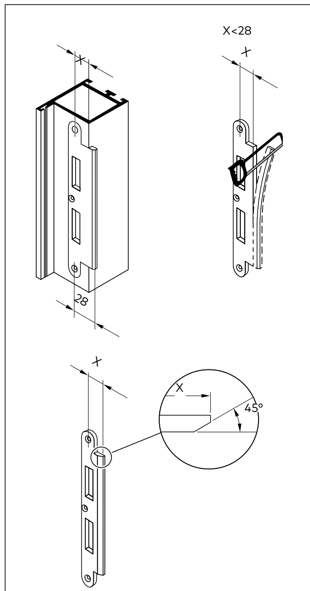
Afb. 19 Maten van de aanpassingen
