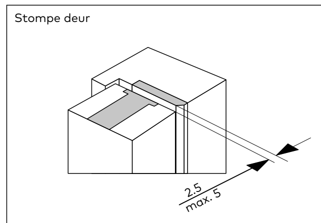
Afb. 32 De deurspleet controleren
