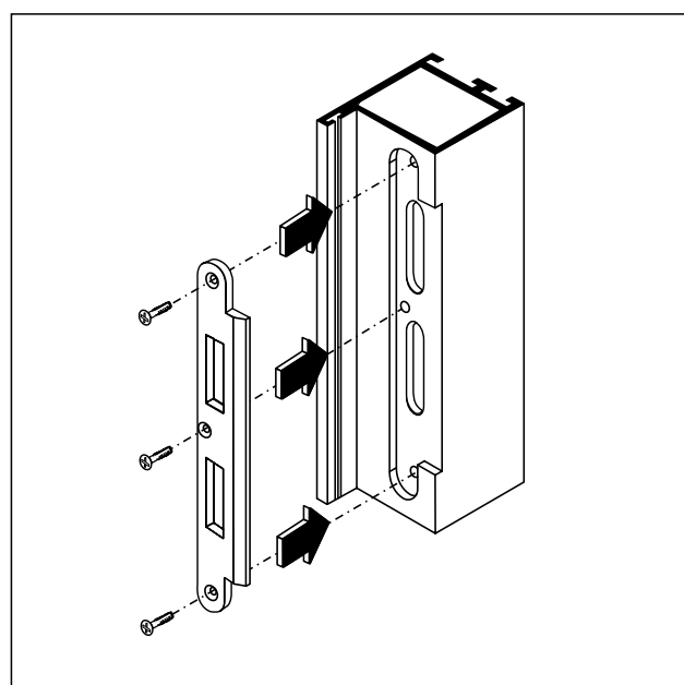
Afb. 20 Monteer de sluitplaat
