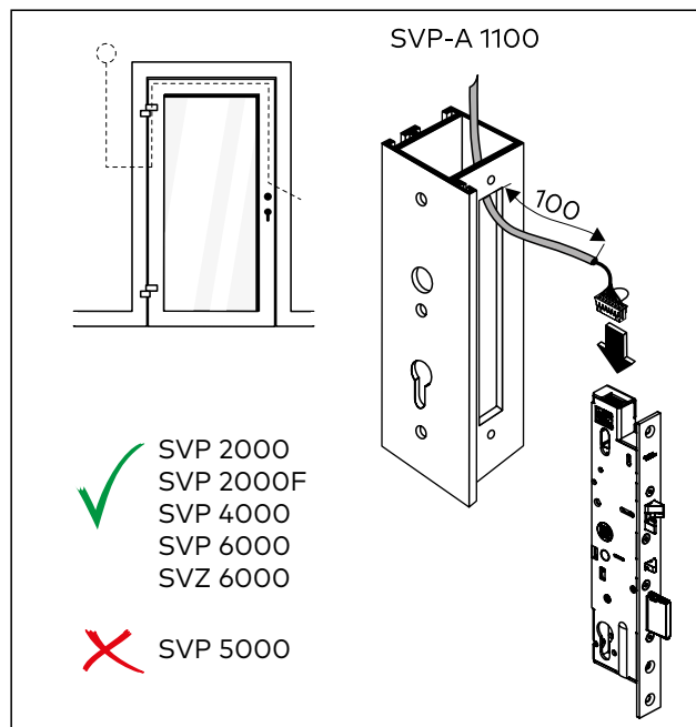
Afb. 15 Kabel aansluiten
