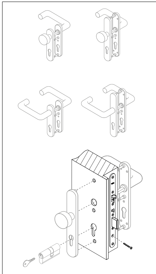
Afb. 25 Monteer de deurkruk en de slotcilinder
