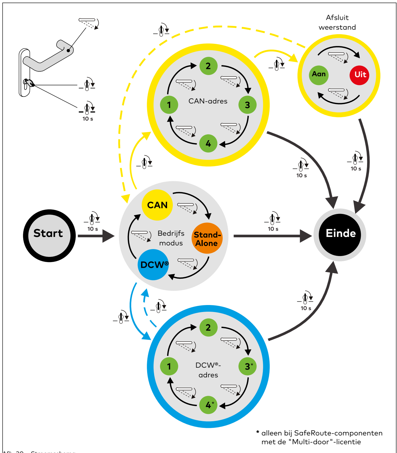
Afb. 30 Stroomschema
