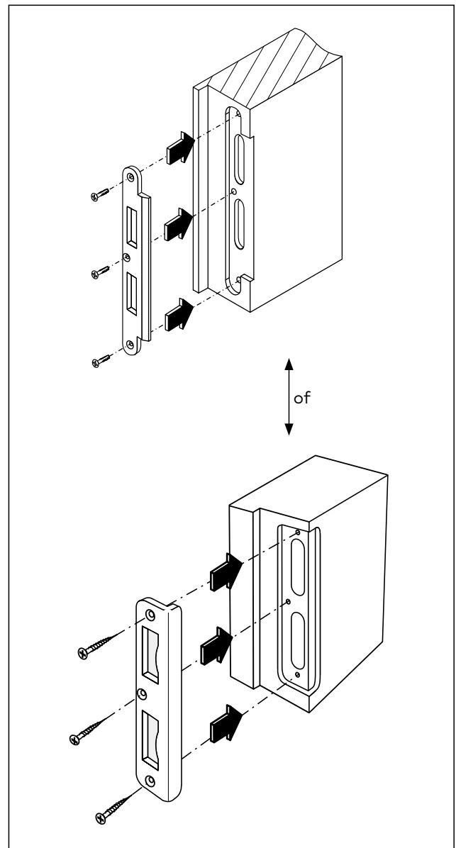
Afb. 27 Monteer de sluitplaat
