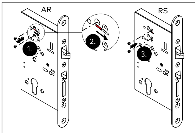
Afb. 21 Werkingsmodus arbeidsstroom naar ruststroom wijzigen
