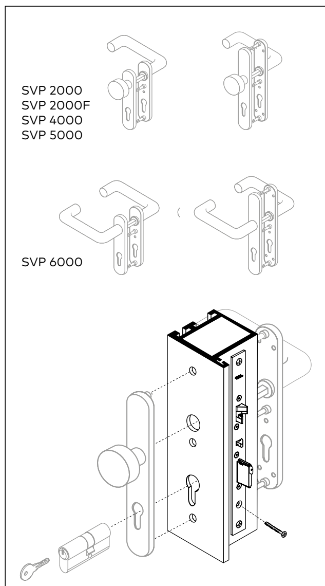
Afb. 18 Monteer de deurkruk en de slotcilinder
