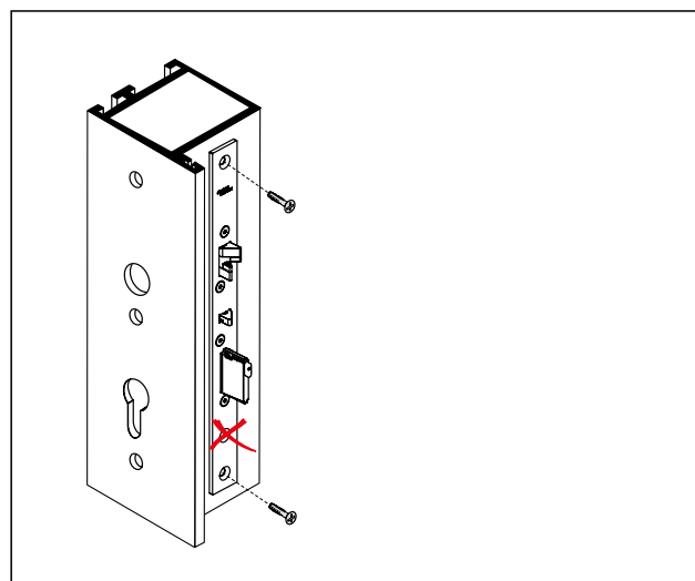
Afb. 17 Anti-paniekslot vastschroeven
