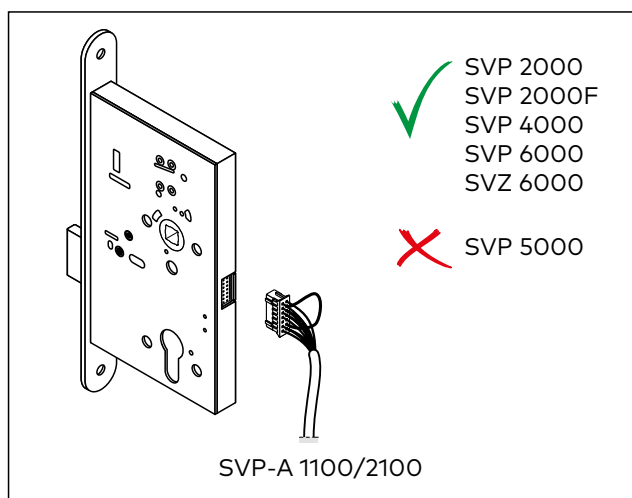
Afb. 22 Kabel aansluiten
