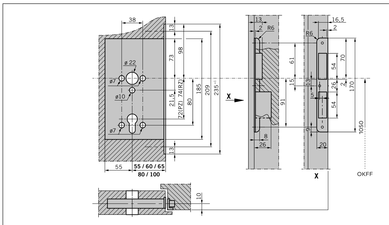
Afb. 12 Uitsparingen en voorgeboorde gaten in het deurblad en het deurkozijn met een hoeksluitplaat
